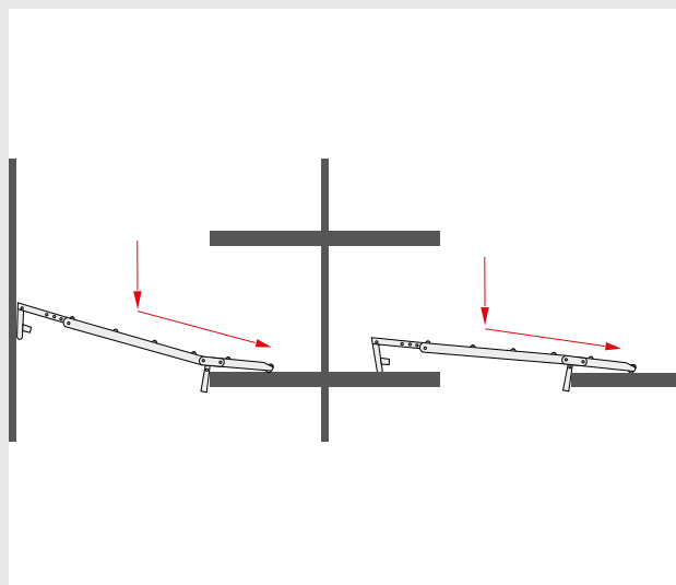
Uso della rulliera RLS in profondità: 1. Vista sezione tomba ipogea: loculi su un lato. 2. Vista sezione tomba ipogea: loculi su entrambi i lati.
